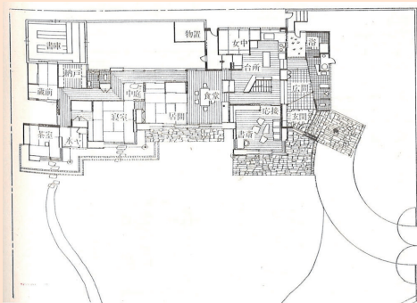
角川邸 平面図 建築文化1956年1月号より転写
