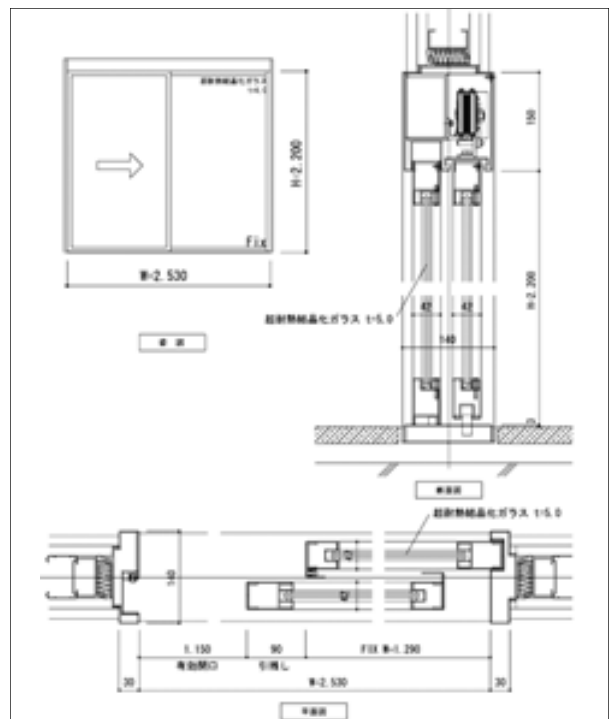
最新認定取得品「手動片引戸フラットレールタイプ」 (W2530ミリ×H2200ミリ、有効開口W1150ミリ)
